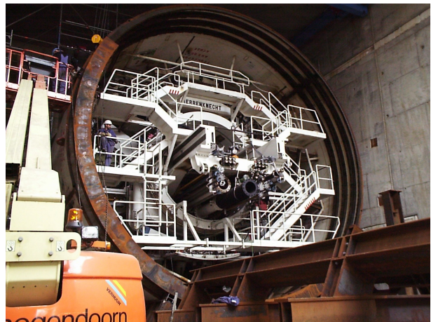
Einbau der Tunnelbohrmaschine
